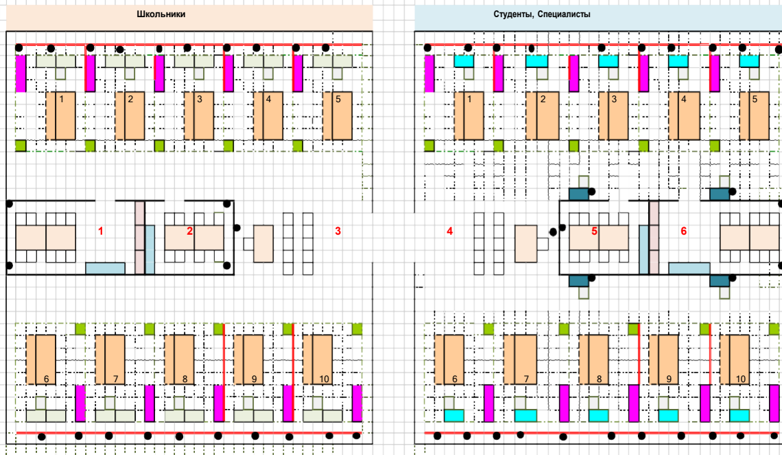
Рекомендуемая схема размещения оборудования на компетенции "ПОРТНОЙ" 40м x 17м. S=680м 2
